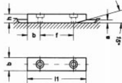
H extremos rectos para 2 tornillos de retención y chafán
