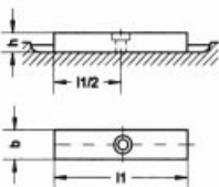
D extremos rectos para tornillo de retención
