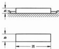
B extremos rectos sin tornillo de retención
