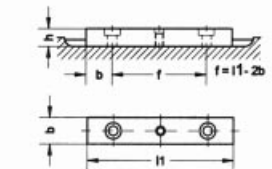
F2) extremos rectos par 2 tornillos de retención y 1 ó 2 torn. de presión
