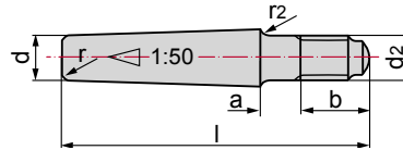
Pasador cónico con espiga roscada y longitudes de espiga constantes
