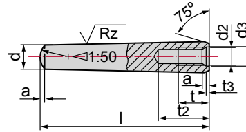
Pasador cónico con rosca interior
