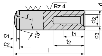
Pasador cilíndrico con rosca interior
